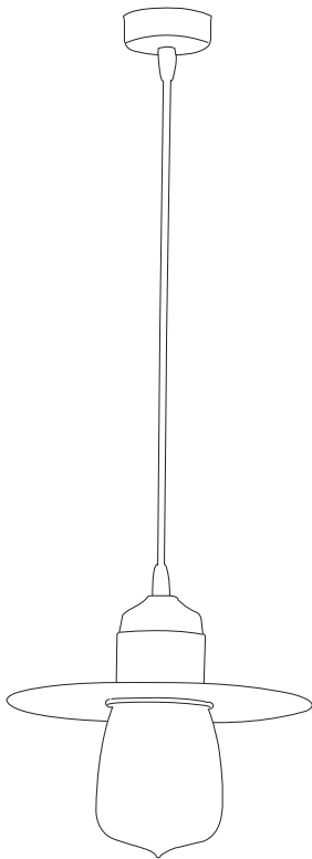
ART. 2956.01 Tutti colori SA - Vetro satinato TR - Vetro trasparente Rosone cm. 8 Disco cm. 28 Totale H. max cm. 150 ART. 2955.01 Foglia oro - argento - rame
