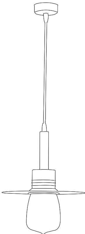
ART. 2967.01 Tutti colori SA - Vetro satinato TR - Vetro trasparente Rosone cm. 8 Disco cm. 28 Totale H. max cm. 150 ART. 2968.01 Foglia oro - argento - rame
