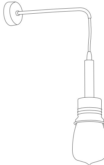
ART. 2970.01 Tutti colori SA - Vetro satinato TR - Vetro trasparente Base cm. 8 Sporgenza cm. 39 Vetro cm. 11,5 Altezza min. cm. 50 Altezza max cm. 150
