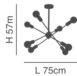
77-8094-56 KQ 2629/8 8xE27, max 60W, 230V
