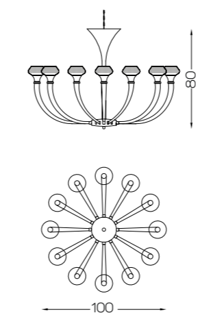
Art. 1946/CH12/NL ø 100 cm H 80 cm 12 x E14 x 40W
