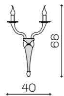
Art 2009/A2 L 40 cm H 66 cm Sp 24 cm 2 x E14 x 40W
