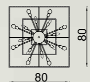
Art. 2022/NL L 80 x 80 cm H 220 cm 16 x E14 x Led 5W
