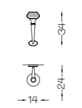
Art. 1946/A1/NL L 14 cm H 34 cm Sp 24 cm 1 x E14 x 40W
