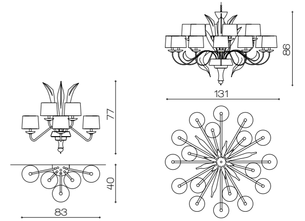
Art. 1930/A5 L 83 cm H 77 cm Pø 18 cm Sp 40 cm 5 x E14 x 25W
