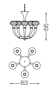
Art. 1946/CH5/NL ø 63 cm H 55 cm 5 x E14 x 40W
