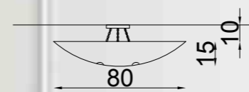
Art. 2101/G/LU Ø 80 cm H 15 cm H tot 25 cm 4 x E27 x Led 7W
