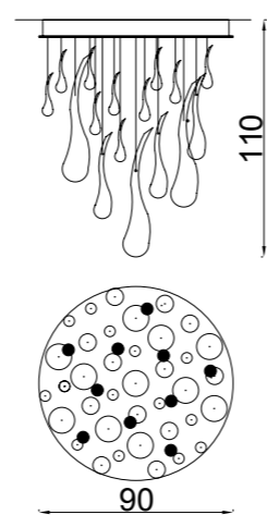
Art. 2063/Steel Ø 90 cm H 110 cm 10 x GU10 x 40W (Available IP65)
