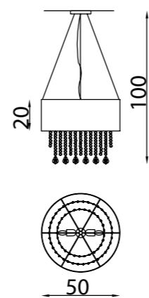
Art. 1386/CH2/NL Pø 50 cm H tot 100cm + 50 cm Steel cable 2 x E27 x 60W
