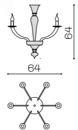
Art 2009/CH6 ø 64 cm H 64 cm 6 x E14 x 40W
