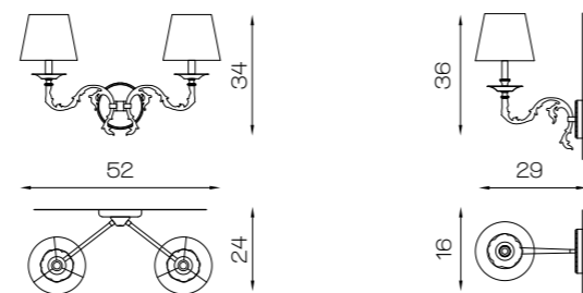
Art. 1986/A2 ø 52 cm H 34 cm Pø 16 cm 2 x E14 x 40W
