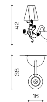
Art. 1631/A1 PØ 16 cm H 42 cm Sp 38 cm 1 x E14 x 40W
