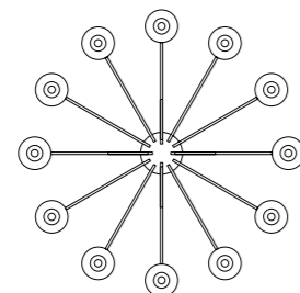
Art. 1742/CH12/KR/V1 ø 132 cm H 90 cm Pø 14 cm 12 x E14 x 25W
