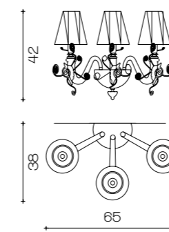
Art. 1631/A3 L 65 cm H 42 cm Sp 38 cm PØ 16 cm 3 x E14 x 40W
