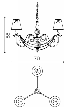
Art. 1794/CH3 Ø 78 cm H 55 cm PØ 16 cm 3 x E14 x 40W
