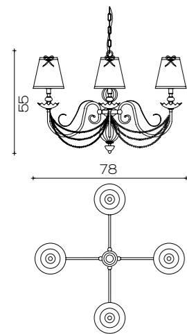
Art. 1794/CH4 Ø 78 cm H 55 cm PØ 16 cm 4 x E14 x 40W
