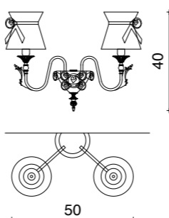
Art. 1850/A2 L 50 cm H 40 cm Sp 28 cm 2 x E14 x 40W
