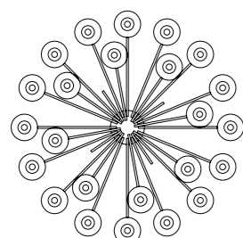
Art. 1742/CH24/KR ø 132 cm H 100 cm Pø 14 cm 24 x E14 x 25W
