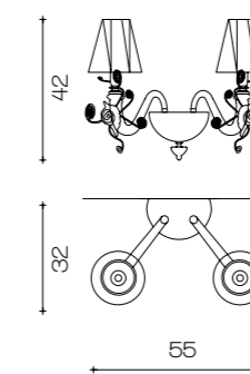
Art. 1631/A2 L 55 cm H 42 cm Sp 32 cm PØ 16 cm 2 x E14 x 40W
