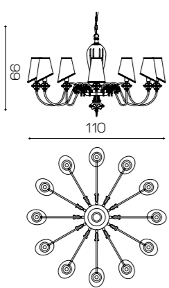
Art. 1774/CH12 ø 110 cm H 66 cm Pø 14 cm 12 x E14 x 40W
