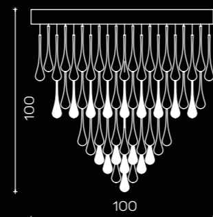
Art. 1615 ø 100 cm H 100 cm 16 x E14 x 60W
