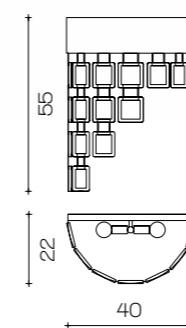
Art. 2174/A L 40 cm H 55 cm Sp 22 cm 2 x E14 x Led
