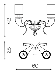
Art. 1770/A1 ø 60 cm H 42 cm Pø 12 cm 2 x E14 x 40W
