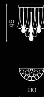
Art. 1359/A H 45 cm L 30 cm 2 x E14 x 40W
