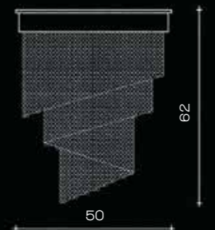
Art. 1537 ø 50 cm H 62 cm 10 x E14 x 60W
