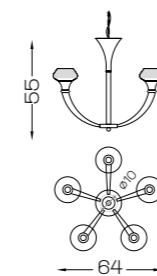
Art. 1946/CH5/NL ø 64 cm H 55 cm 5 x E14 x 40W
