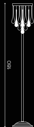
Art. 1359/FL ø 30 cm H 180 cm 3 x E14 x 40W
