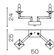
Art. 2032/A2/NL L 50 x 25 cm H 24 cm 2 x E14 x 40W
