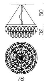
Art. 2082/NL ø 78 cm H 32 cm +50 cm steel cable 8 x E14 x 40W
