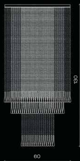
Art. 1536 ø 60 cm H 130 cm 12 x E14 x 60W
