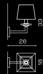
Art. 1214 Speciale A1 P lato 18 cm L 26 cm H 33 cm Sp 26 cm 1 x E27 x 40W
