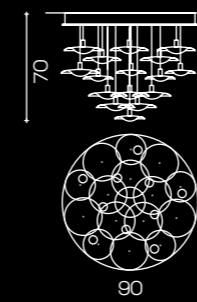
Art. 2060/Steel ø 90 cm H 70 cm 10 x GU10 x 40W (Available IP65)
