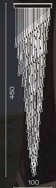
Art. 1810 Ø 100 cm H 450 cm 40 x E14 x 25W
