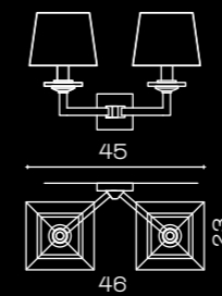
Art. 1214 Speciale A2 P lato 18 cm L 46 cm H 33 cm Sp 23 cm 2 x E27 x 60W
