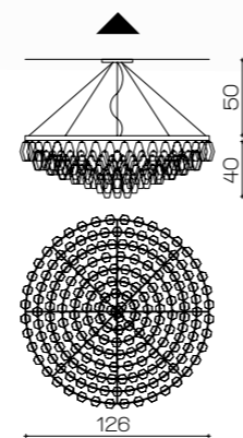
Art. 2081/NL ø 126 cm H 40 cm 50 Kg +50 cm Steel cable 16 x E14 x 40W
