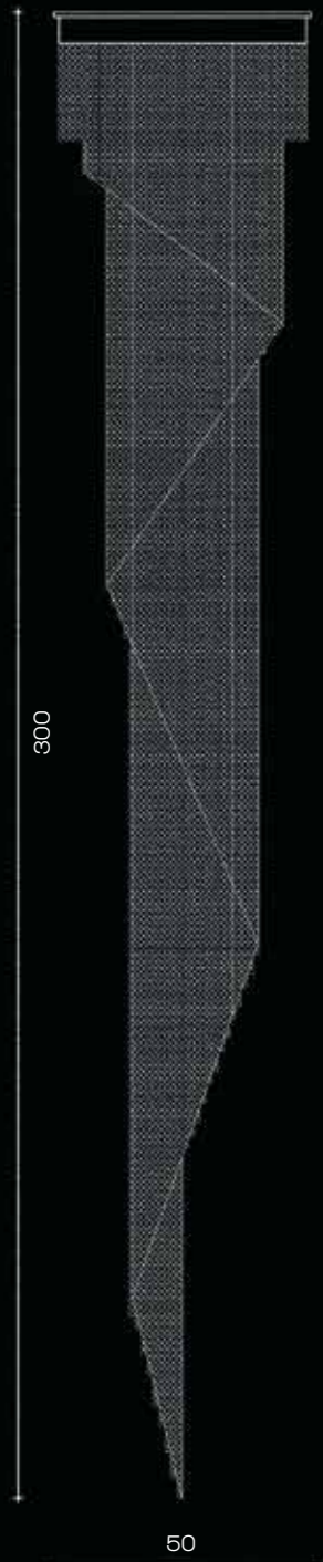
Art. 1379 ø 50 cm H 300 cm 12 x E14 x 60W
