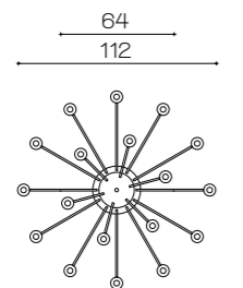
Art. 2009/CH18 ø 112 cm H 112 cm 18 x E14 x 40W
