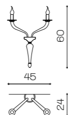
Art. 2009/A2 L 45 cm H 60 cm Sp 24 cm 2 x E14 x 40W
