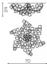
Art. 2171/Ceiling/G ø 70 cm H 24 cm 6 x E14 x Led
