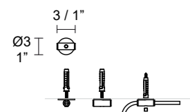
Kit decentramento Decentralization kit
