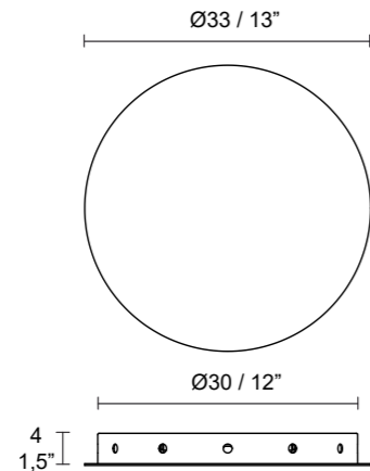
Rosone decentramento 12 Canopies Decentralization 12
