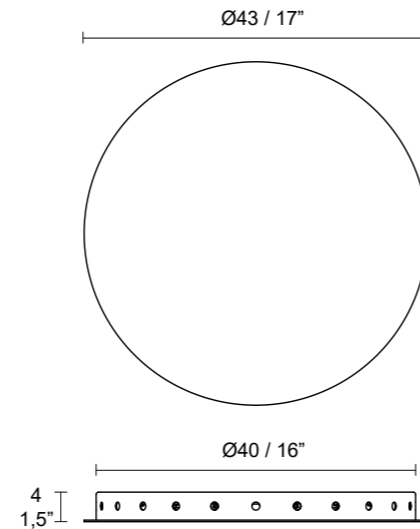
Rosone decentramento 24 Canopies Decentralization 24
