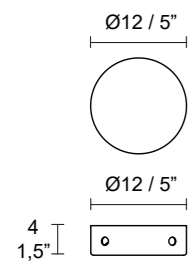
Rosone decentramento 1/4 Canopies Decentralization 1/4
