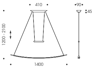
LISGO SKY | LISGO SKY SHORT
