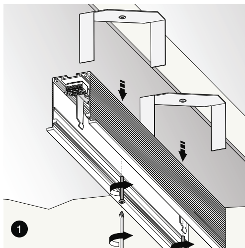
XM2038/39-U Giunzione lineare Linear junction
