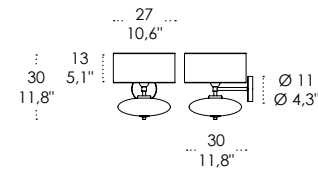
LSH23 E27 ELLISSE / ELLIPSE
