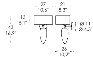
LSH22 E27 OGIVA / OGIVE
