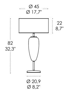
LSH06 E27 OGIVA / OGIVE
