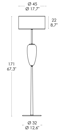
LSH12 E27 OGIVA / OGIVE
