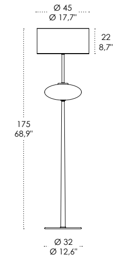
LSH13 E27 ELLISSE / ELLIPSE
