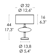
LSH03 E27 ELLISSE / ELLIPSE
